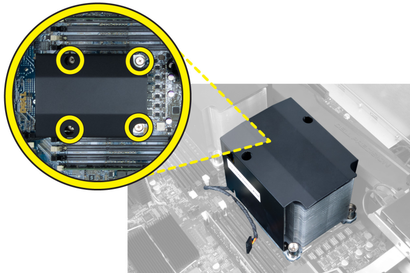
5. הרים את גוף הקירור והסר אותו מהמחשב.
