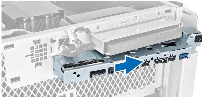
7. הסר את הברגים שמהדקים את מודול ה-USB 3.0 ללוח הקלט/פלט הקדמי והסר אותו מהמחשב.
