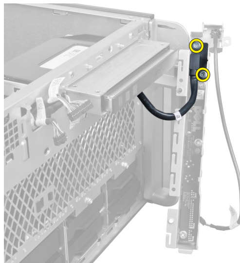
8. הסר את הברגים שמהדקים את לוח הקלט/פלט הקדמי והסר אותו מהמחשב.
