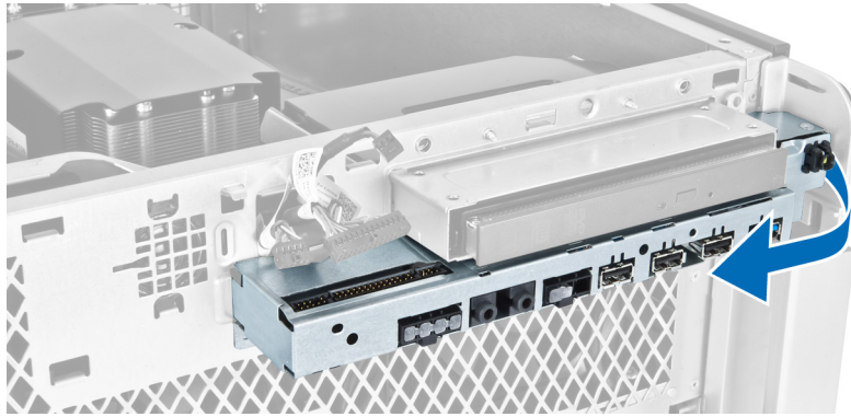
6. החלק את הקצה הנגדי של לוח הקלט/פלט הקדמי כלפי חוץ כדי לנתק את מודול הקלט/פלט מהמארז.
